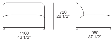
elemento centrale/central unit
